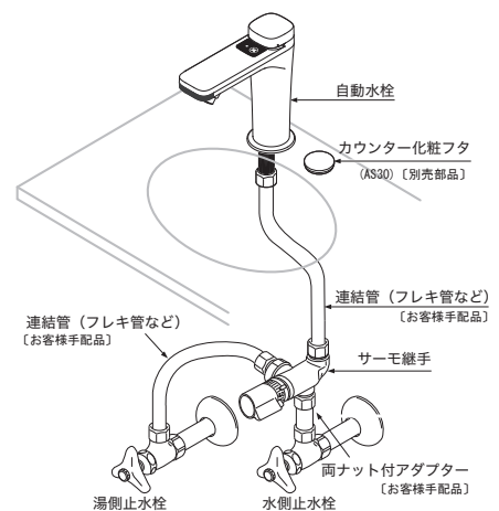
接続例 (台付き 2 ホール混合水栓からの交換)
